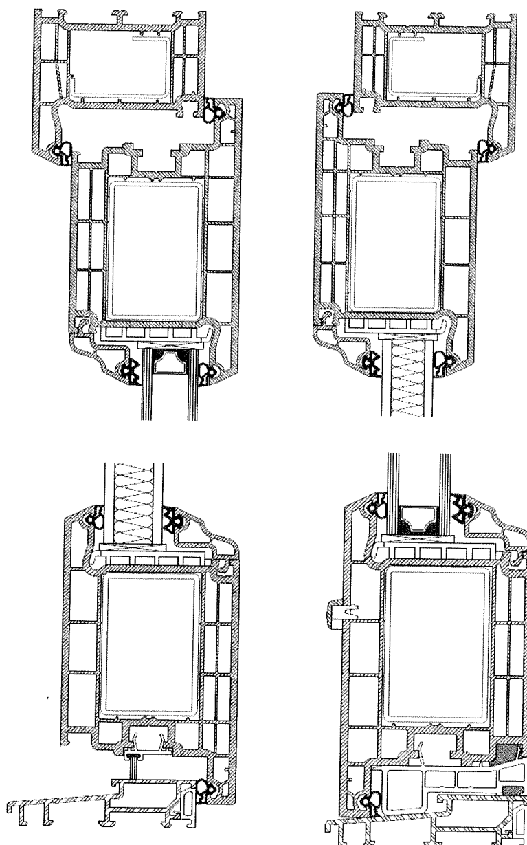
Obrázek 1 – Řez dveřmi
